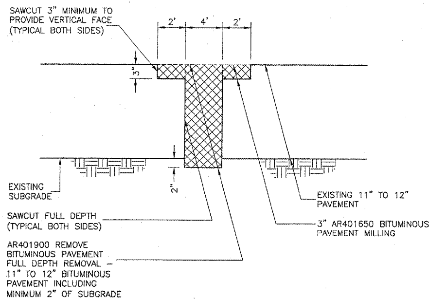
REMOVAL SECTION N.T.S.
