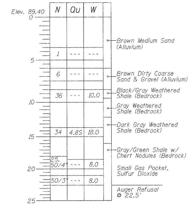
BORING B-4 STA 120+40 (Prop.), 0' Lt.
