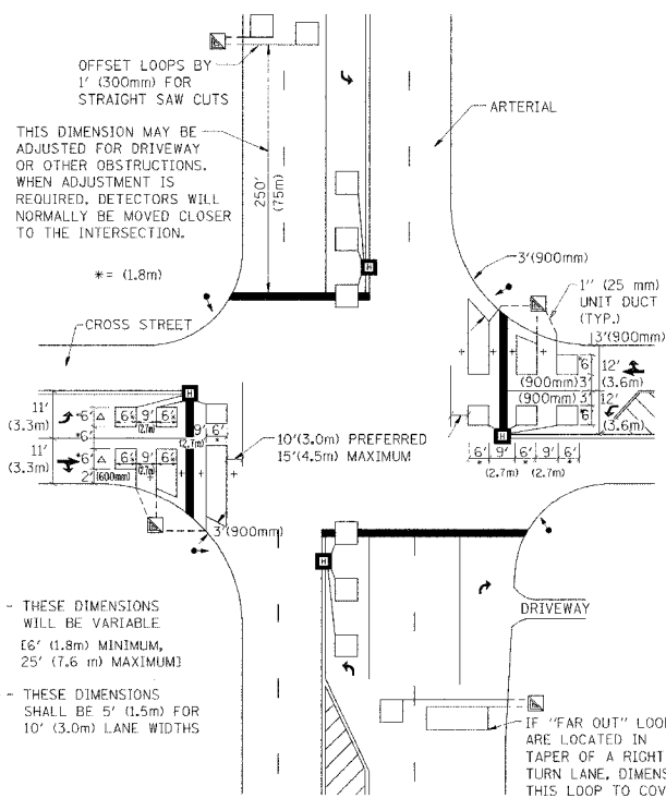
DETAIL 2 N.T.S.
