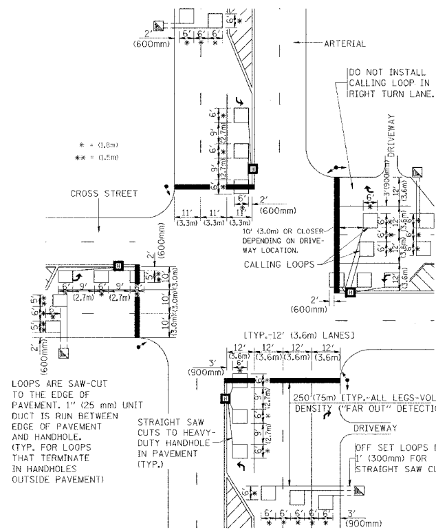
DETAIL 1 N.T.S.
