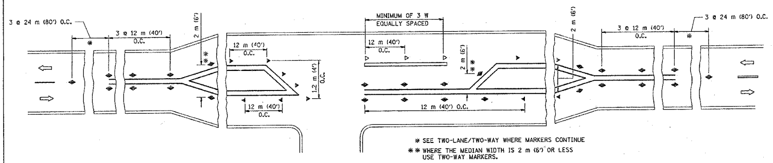
LEFT TURN
