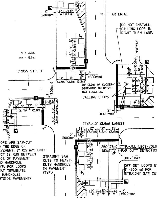
DETAIL 1 N.T.S.
