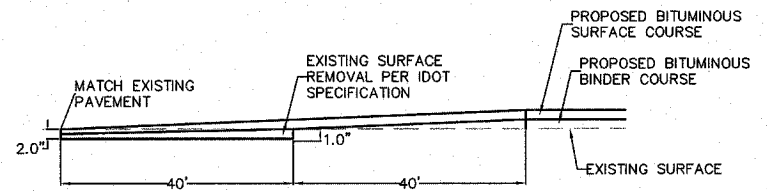
BUTT JOINT DETAIL (STA. 206+79.85 TO STA. 207+59.85 STA. 224+55.51 TO STA. 225+35.51 STA. 226+64.42 TO STA. 227+44.42)
