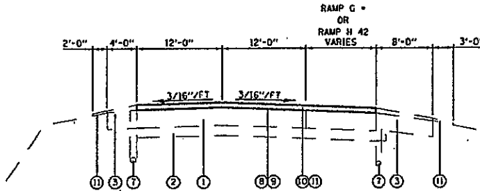
TYPICAL SECTION N.B. 203 STA. 130+50 TO STA. 134+04 •• S.B. 203 STA. 125+21 TO STA. 131+00 •
