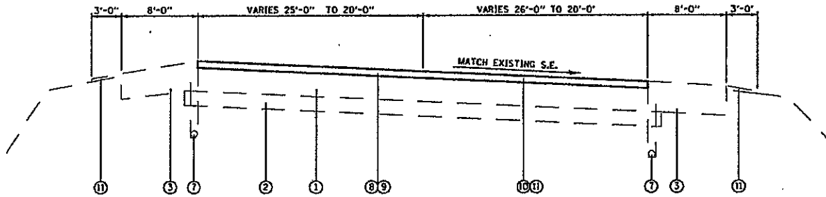
TYPICAL SECTION IL 203 STA. 196+07 TO 200+12
