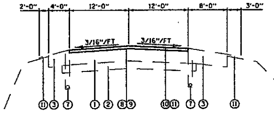
TYPICAL SECTION N.B. 203 STA. 109+50 TO STA. 121+48
