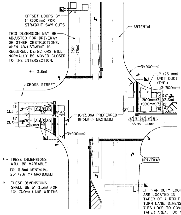
DETAIL 2 N.T.S.
