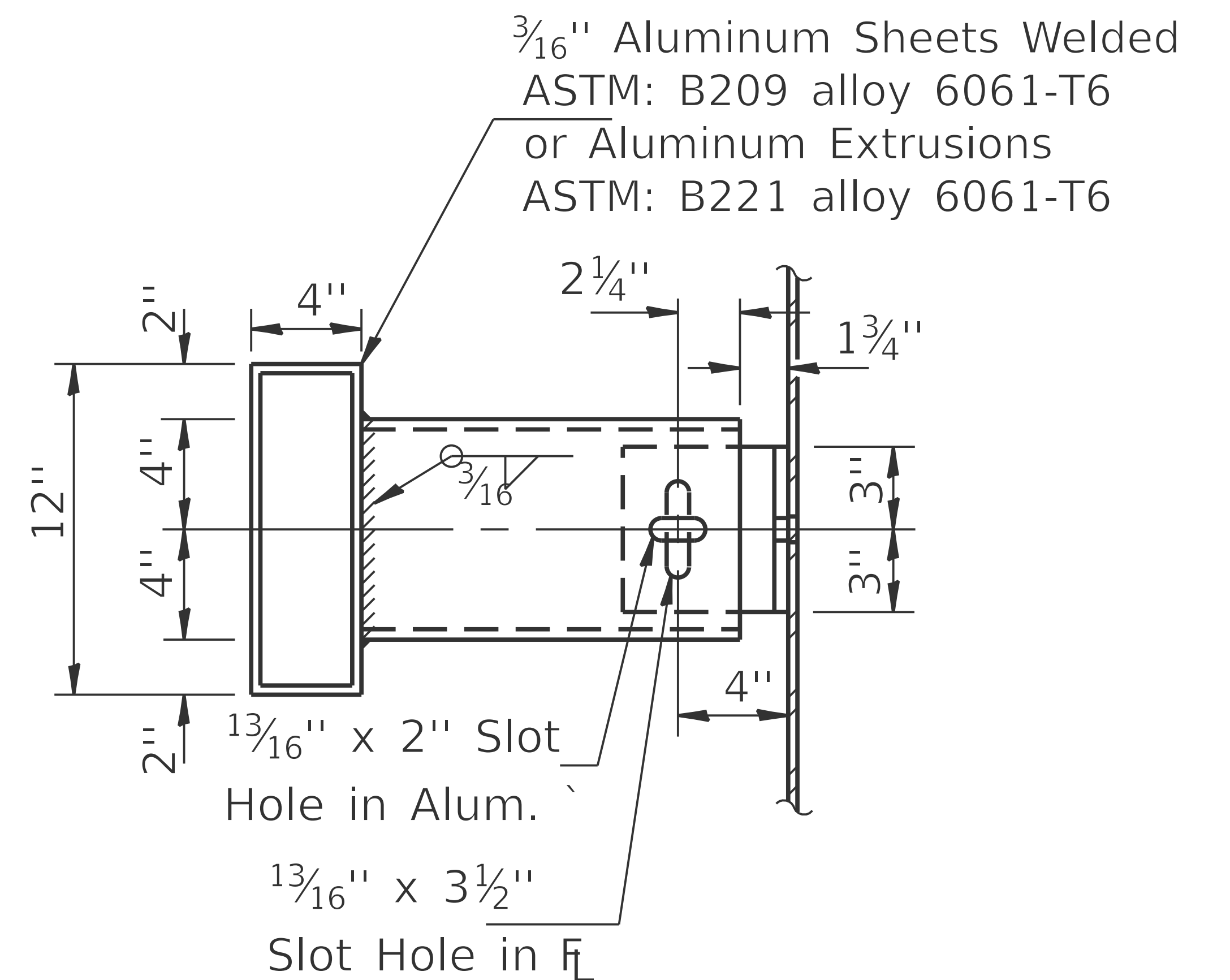
SECTION A-A
