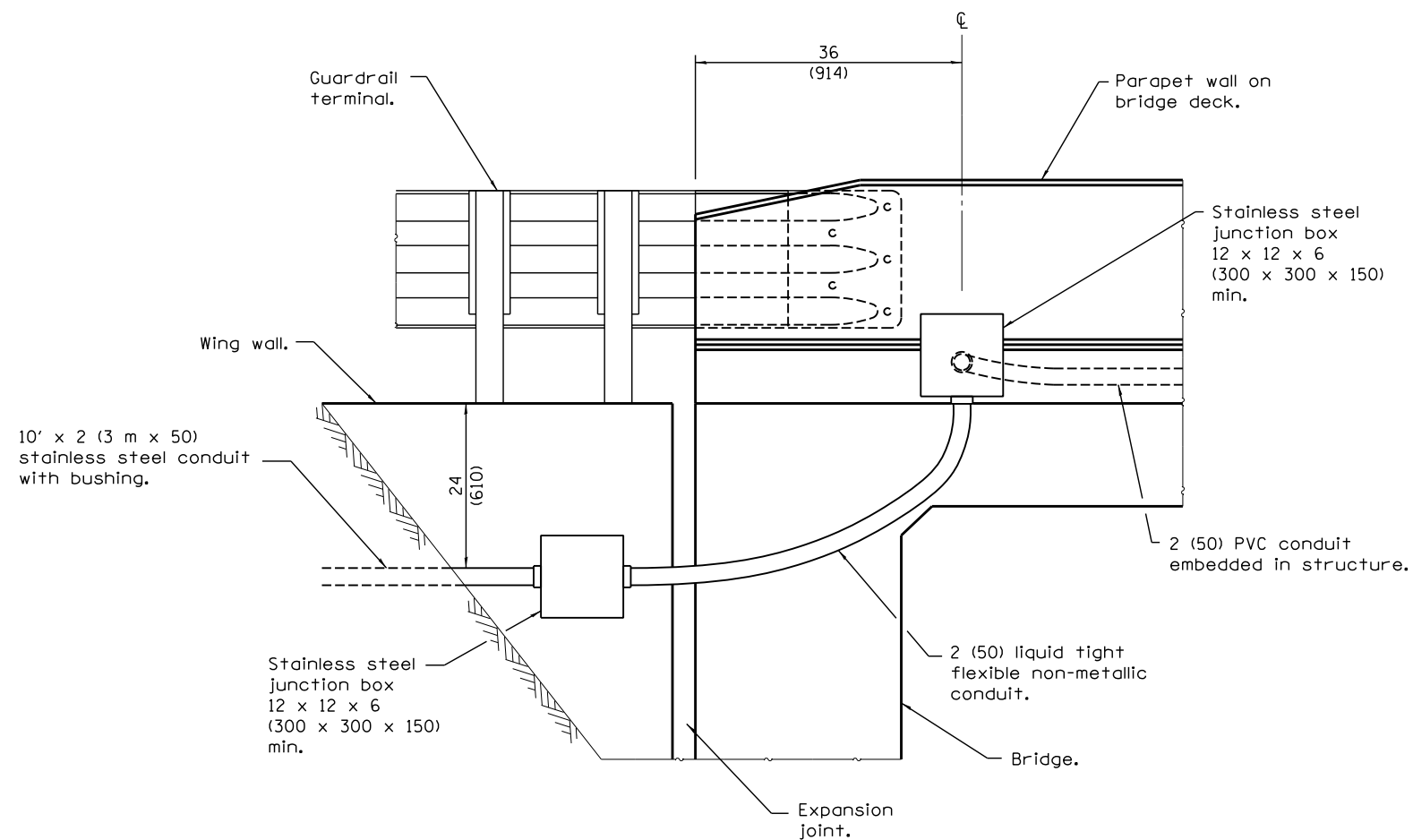
ELEVATION
