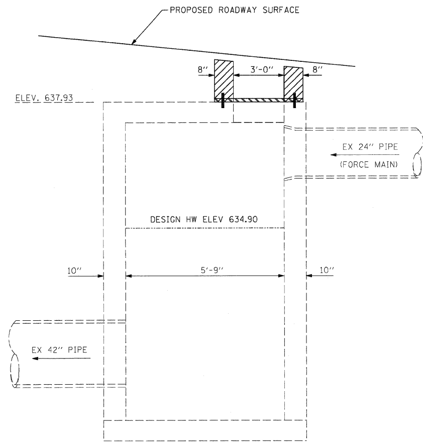
B-B
