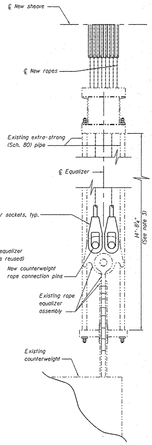
VIEW A-A
