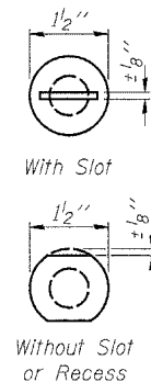
VIEW A-A
