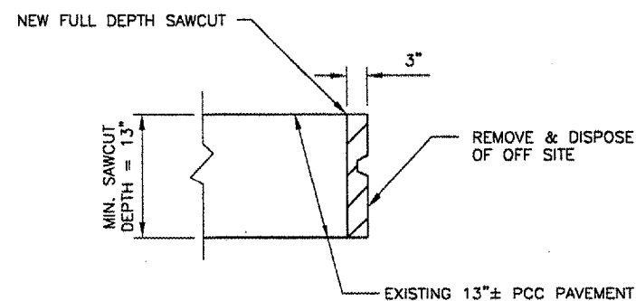
PCC PAVEMENT EDGE SAWING DETAIL N.T.S.
