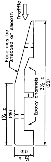
SECTION A-A
