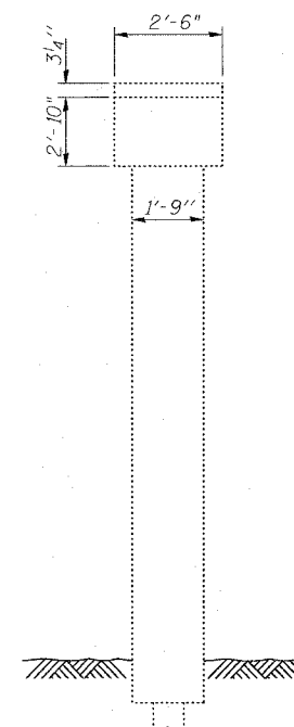
END ELEVATION
