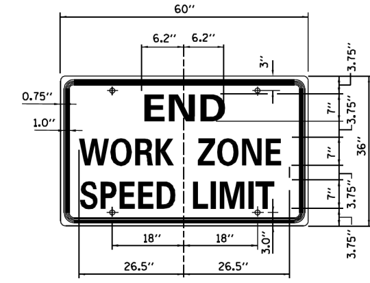
SIGN G20-I103 (O)
