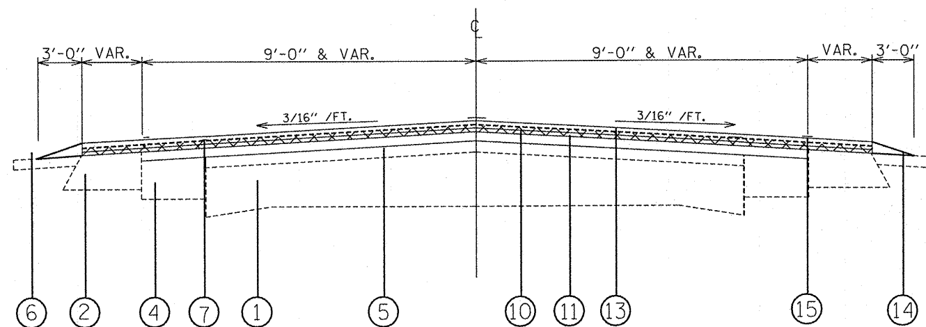
TYPICAL SECTION NO. 6 STA. 136+46.6 TO STA. 137+71 (RT.) STA. 136+43.3 TO STA. 137+71 (LT.)
