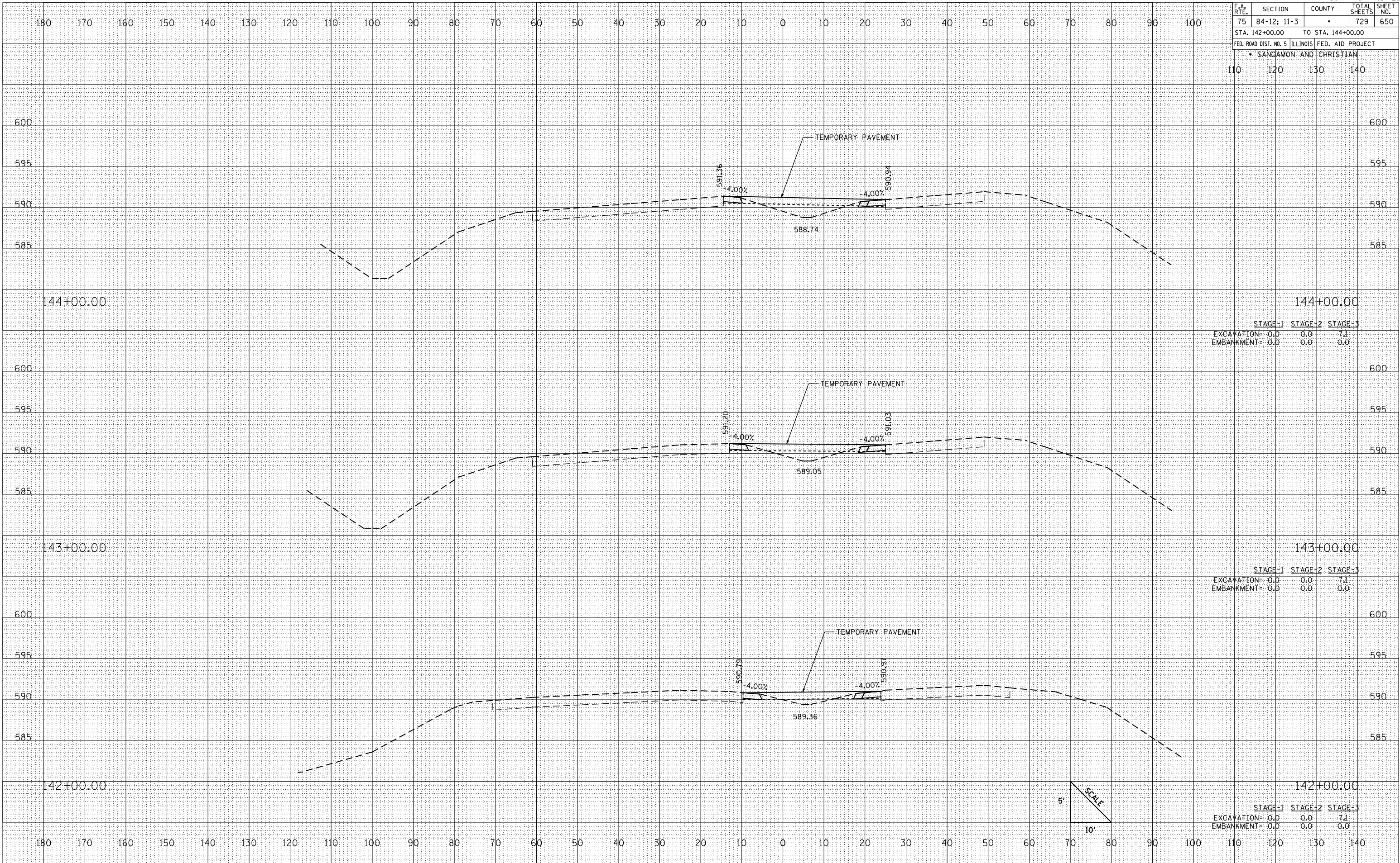
CROSS SECTIONS: IL RTE. 29 – STA. 142+00 TO STA. 144+00
