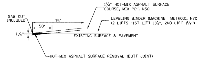
BUTT JOINT DETAIL STA 20+30 TO STA 21+05 & STA 30+90 TO STA 31+65
