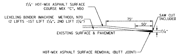
BUTT JOINT DETAIL STA 16+50 TO STA 17+25 & STA 28+95 TO STA 29+70
