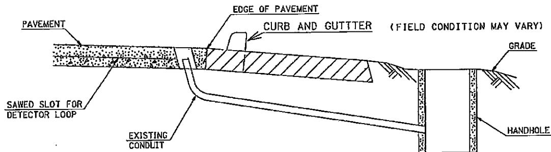
DETAIL (NO SCALE)
