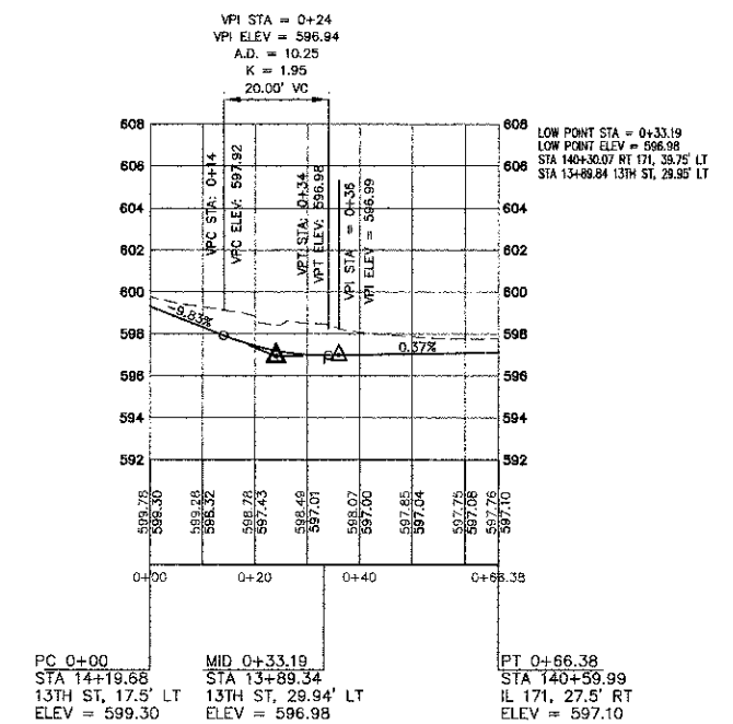
NE PROFILE
