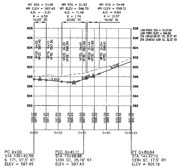
SE PROFILE
