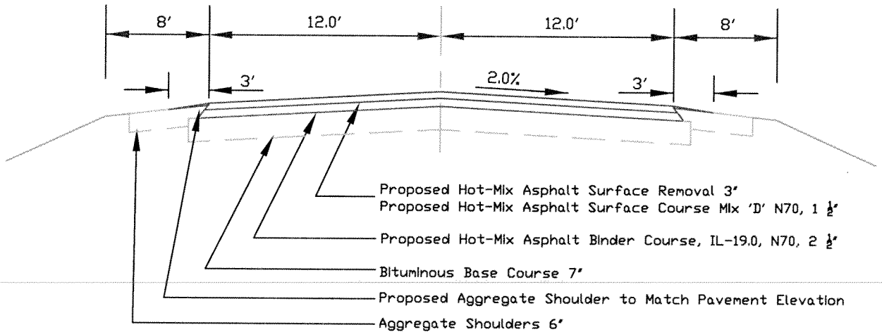
PROPOSED TYPICAL SECTION STA. 26+67.30 TO STA. 40+03.30 STA. 40+97.30 TO STA. 108+35.10 STA. 110+40.60 TO STA. 152+31.00
