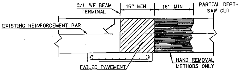
SECTION D-D
