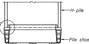
ELEVATION
