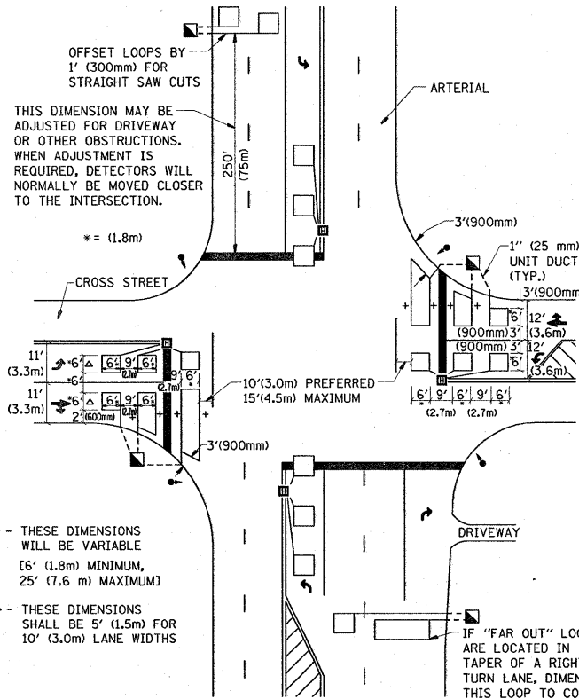
DETAIL 2 N.T.S.
