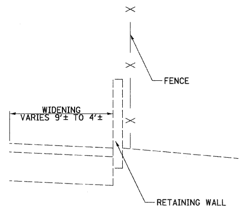
DETAIL A STA. 101+66± TO STA. 102+81±
