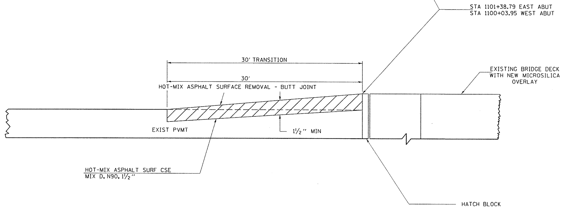
SECTION A-A
