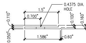
G2 SECTION - TILE SCALE : 1:1
