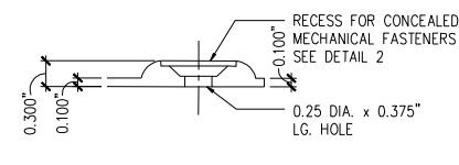
G5 SECTION - TILE SCALE : 1:1
