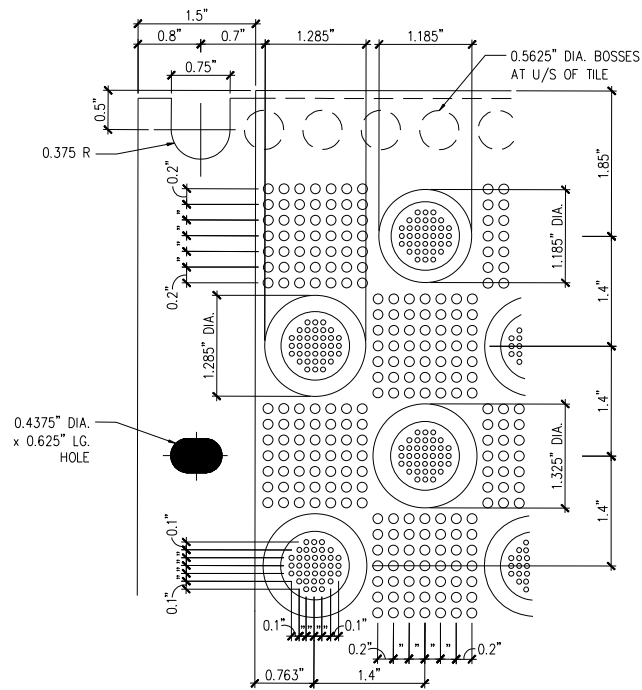
E2 PLAN DETAIL - TILE SCALE : 1:1
