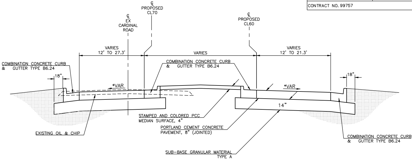
TO BE USED STA 62+16.60 TO STA 63+76.42 (CL60)
