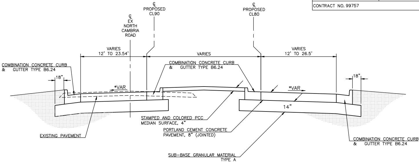
TO BE USED STA 82+00.24 TO STA 83+76.73 (CL80)
