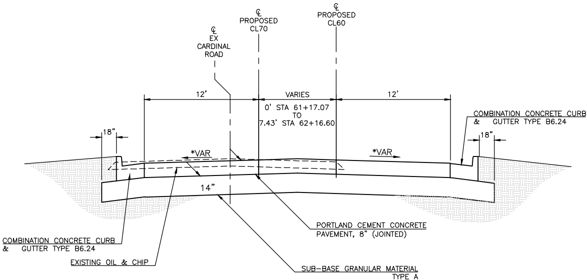
TO BE USED STA 61+17.07 TO STA 62+16.60 (CL60)
