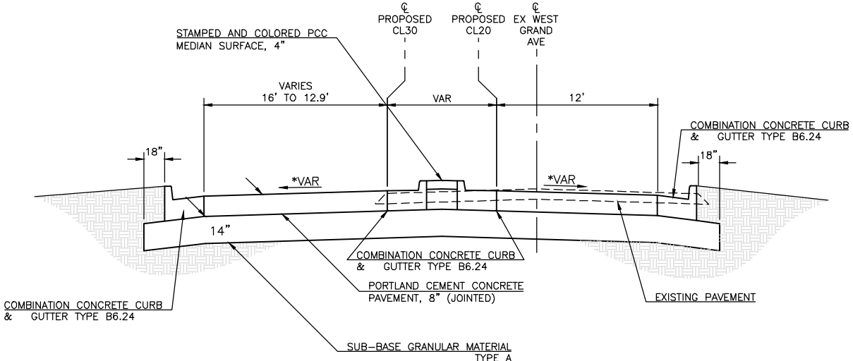
TO BE USED STA 20+74.30 TO STA 21+02.91 (CL20)
