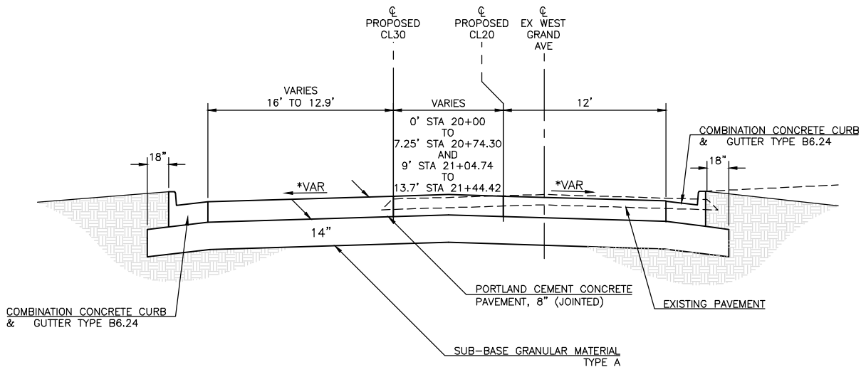
TO BE USED STA 20+00 TO STA 20+74.30 (CL20) STA 21+04.74 TO STA 21+44.42 (CL20)
