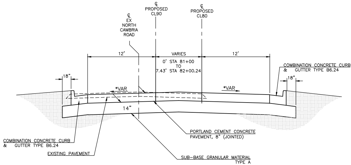
TO BE USED STA 81+00 TO STA 82+00.24 (CL80)
