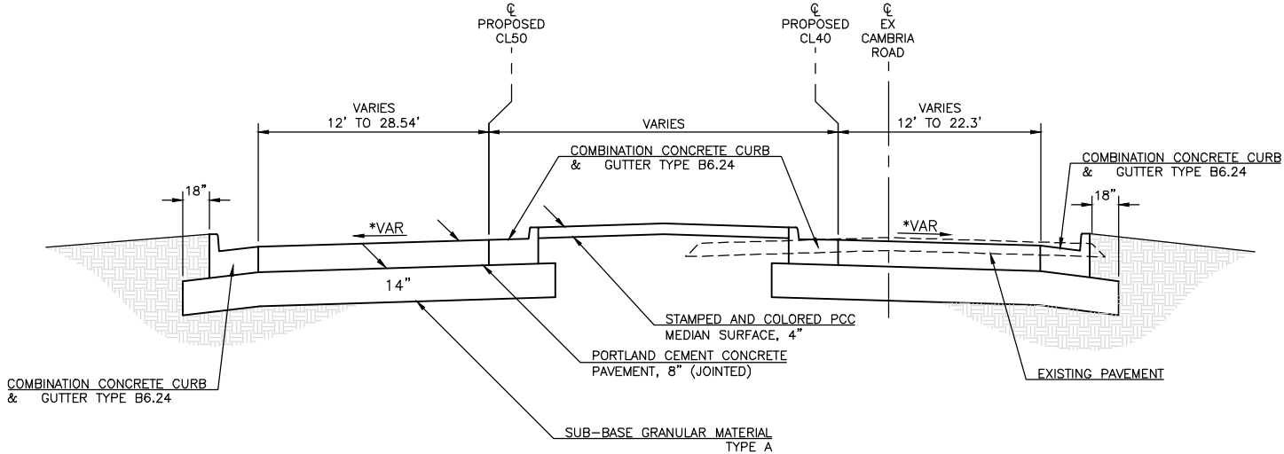
TO BE USED STA 51+43.01 TO STA 53+32.19 (CL50)
