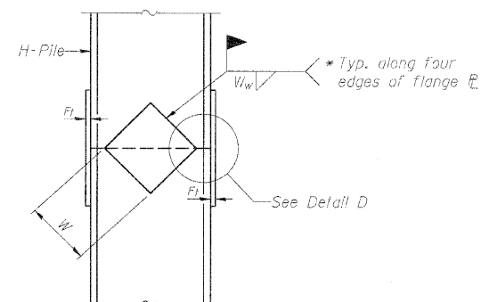
PILE ENCASEMENT
