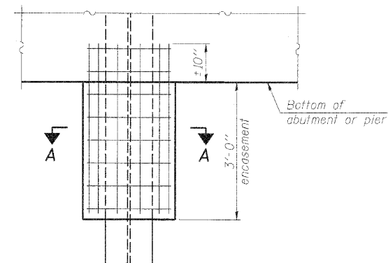
PILE ENCASEMENT
