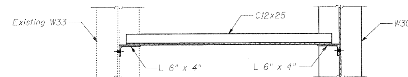
SECTION D-D
