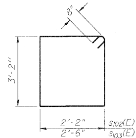
BARS S102(E) & S103(E)
