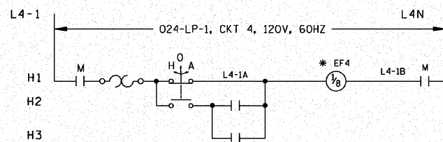
STAIRWELL EXHAUST FAN EF-4
