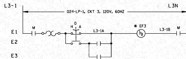
TRASHRACK ROOM EXHAUST FAN EF-3
