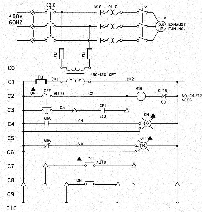
ELECTRICAL ROOM EXHAUST FAN EF-1
