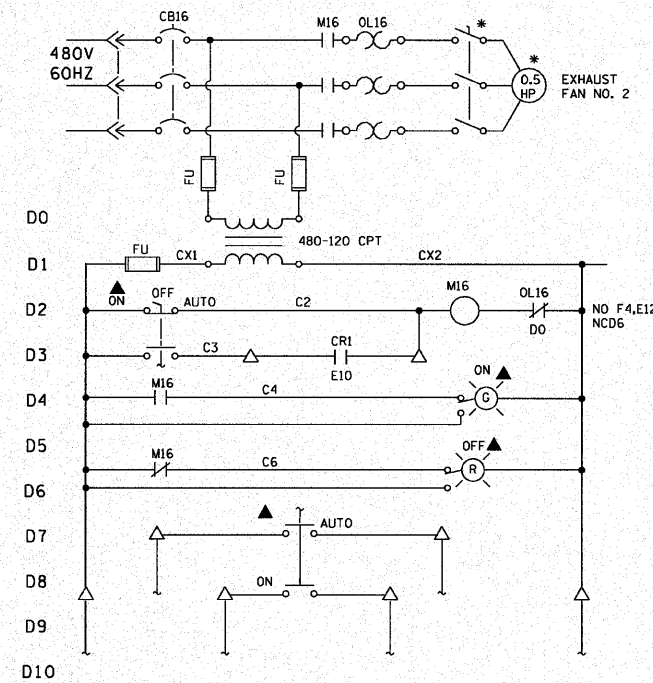
PUMP ROOM EXHAUST FAN EF-2
