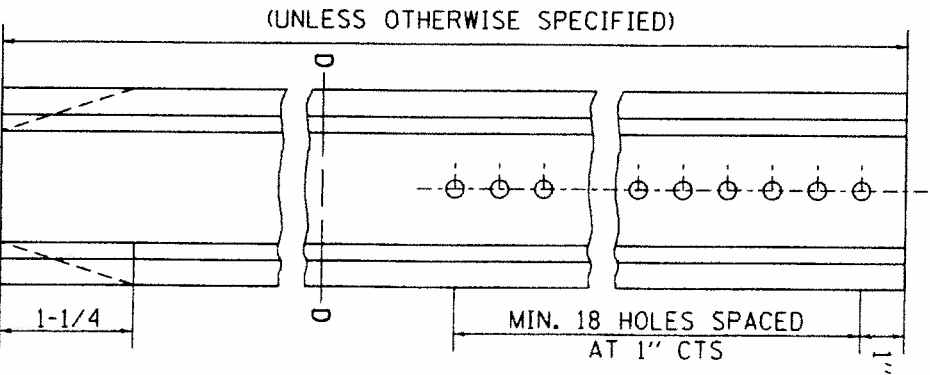
SECTION D-D
