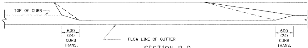
SECTION D-D
