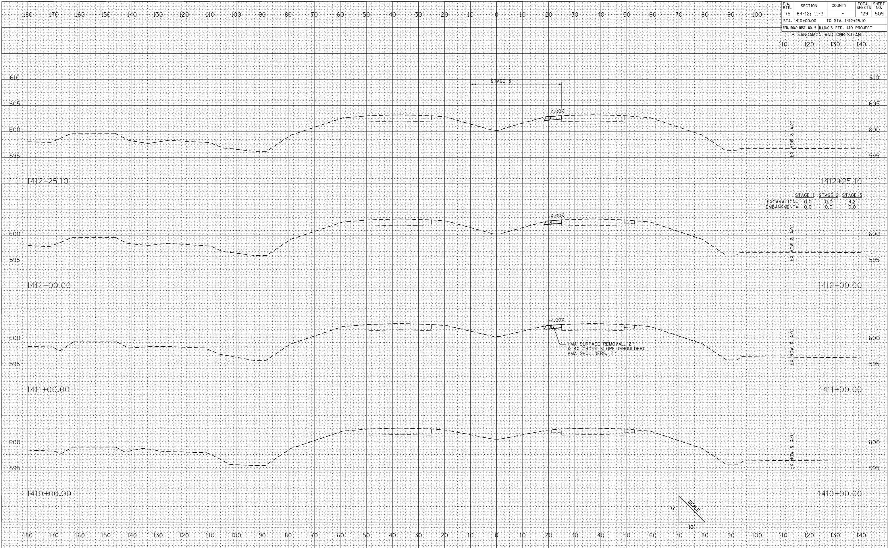
CROSS SECTIONS: IL RTE. 29 – STA. 1410+00 TO STA. 1412+25.10
