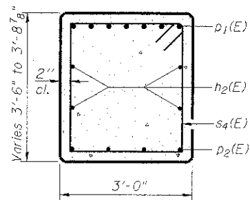
SEC. A-A
