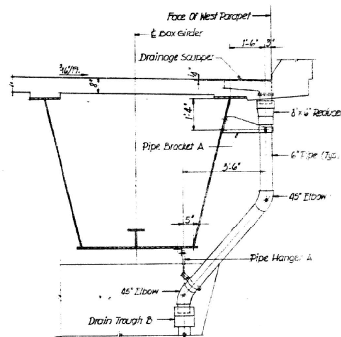
SECTION D-D
