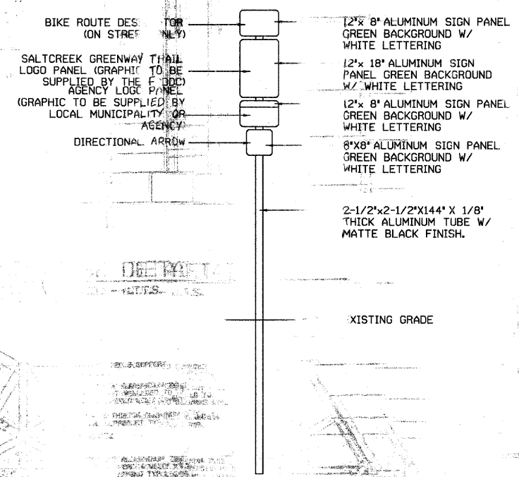
TRAIL MARKER ELEVATION - N.T.S.
